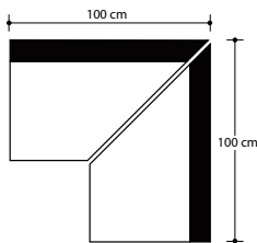
Außenecke: 2-teilig
